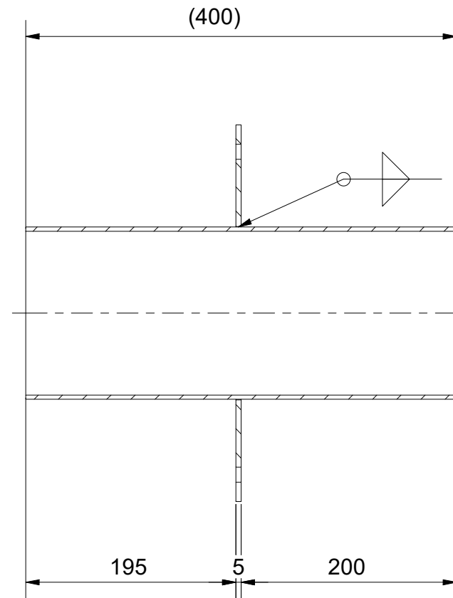
A-A ( 1 : 5 )
